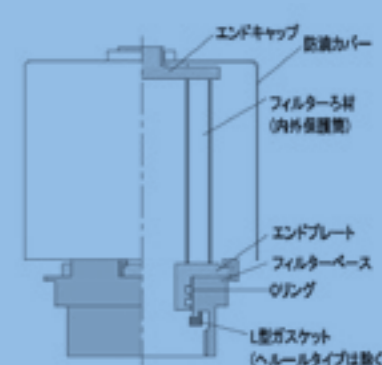
構造図 (VCP-400型)
